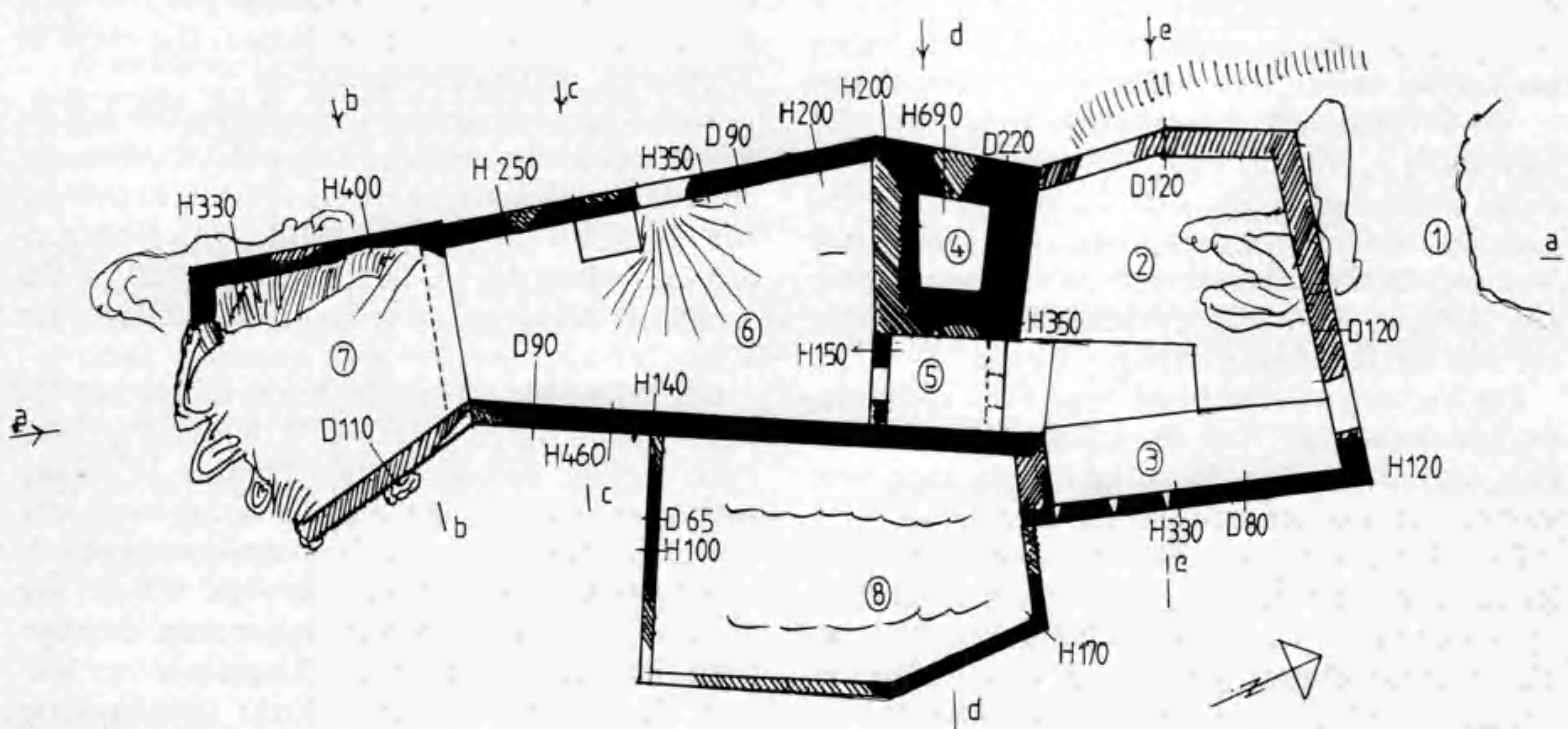
Grundriß der Burgruine Schatzberg
